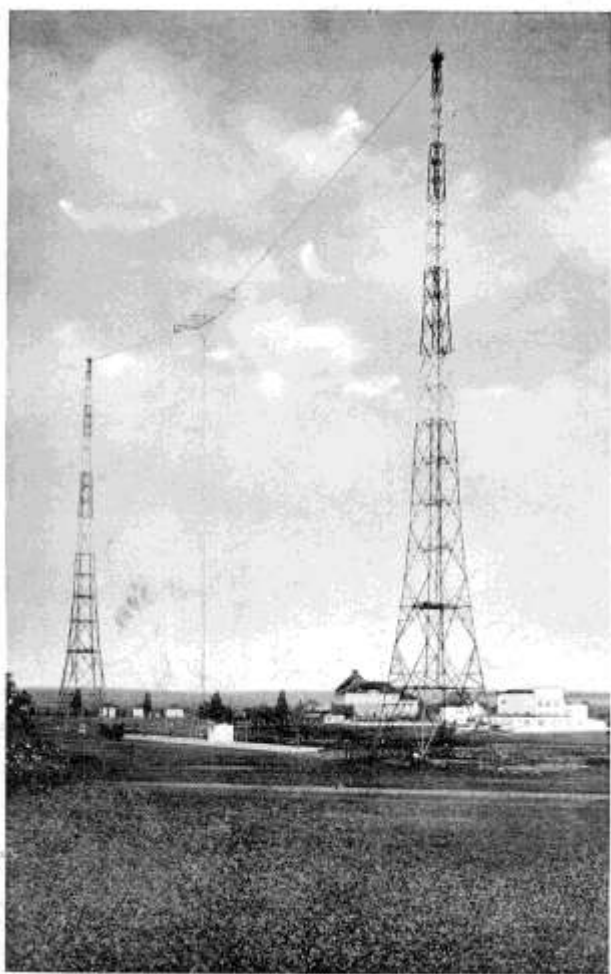
Vysílací stanice čsl. rozhlasu v Liblicích u Ces. Brodu.
